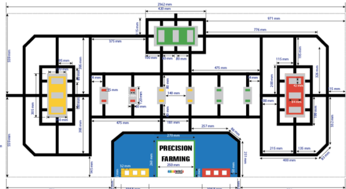
《中学生の部》 コース配置例
