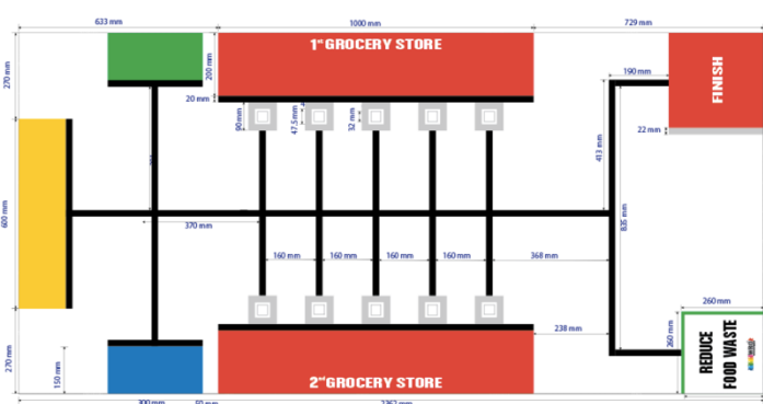
《小学生の部》 コース配置例
